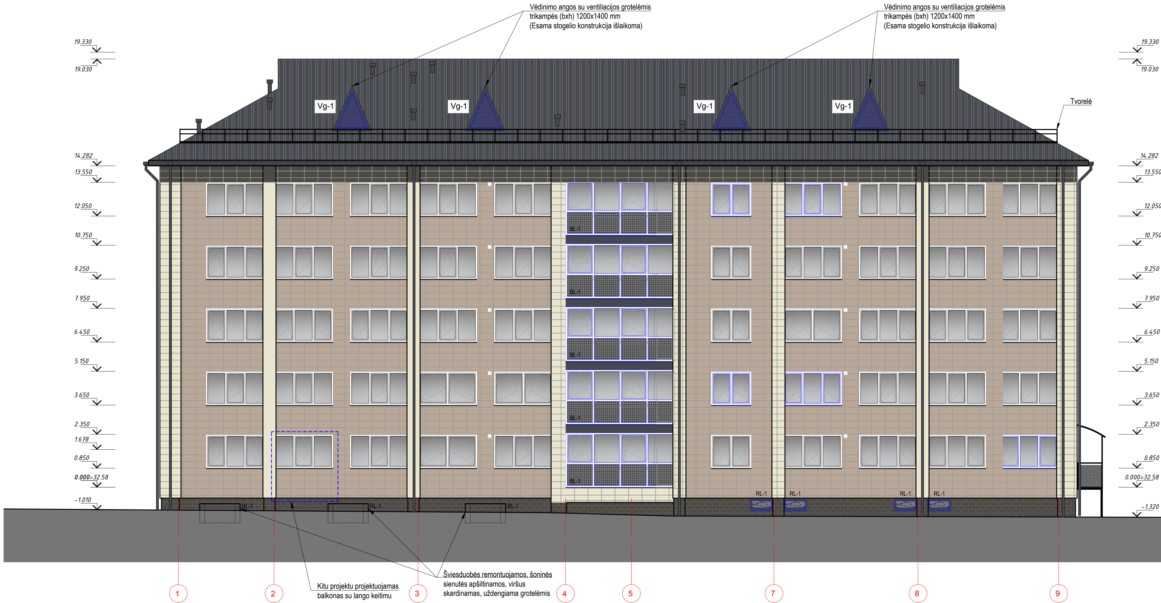
FASADAS 1-9 M 1:100
