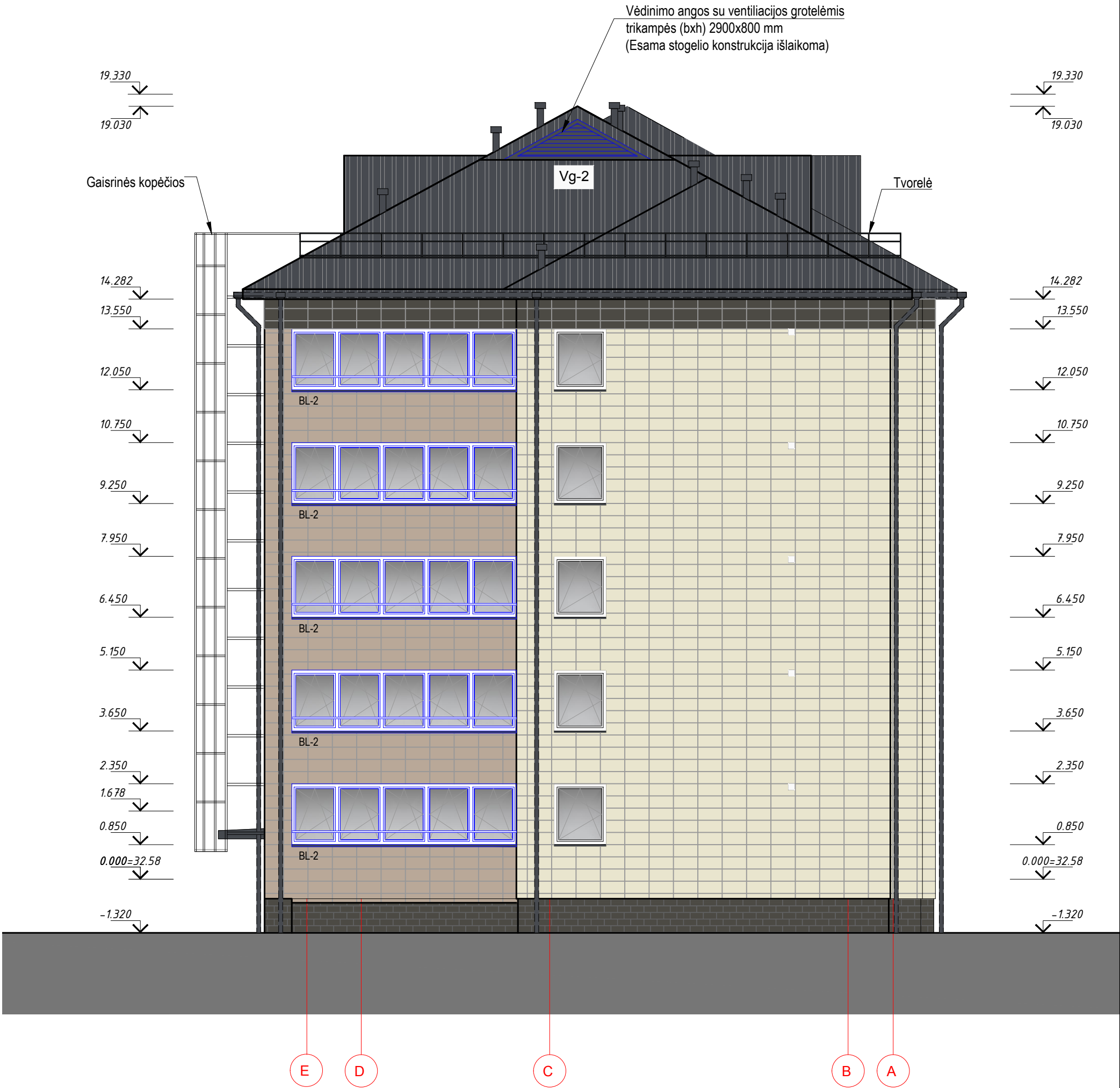
FASADAS E-A M 1:100
