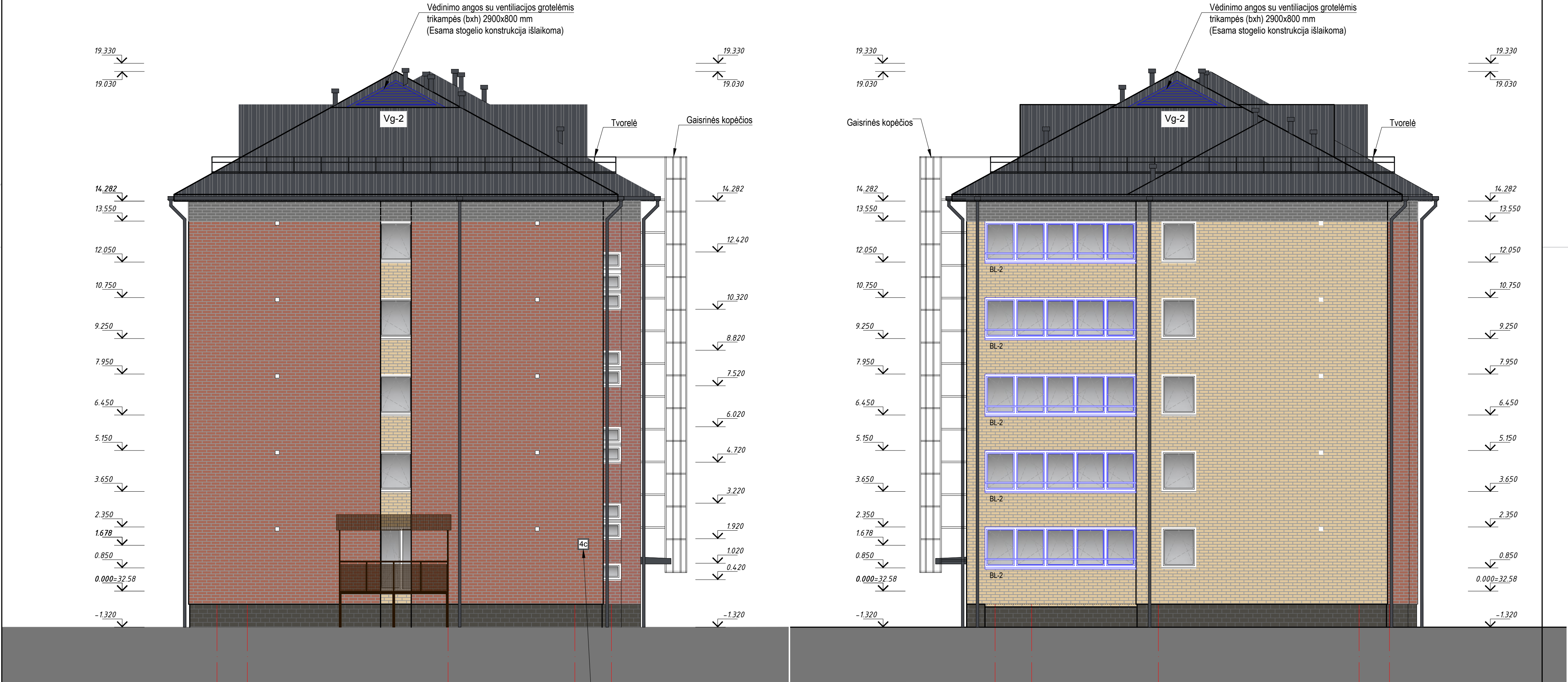
FASADAS A-E M 1:100
