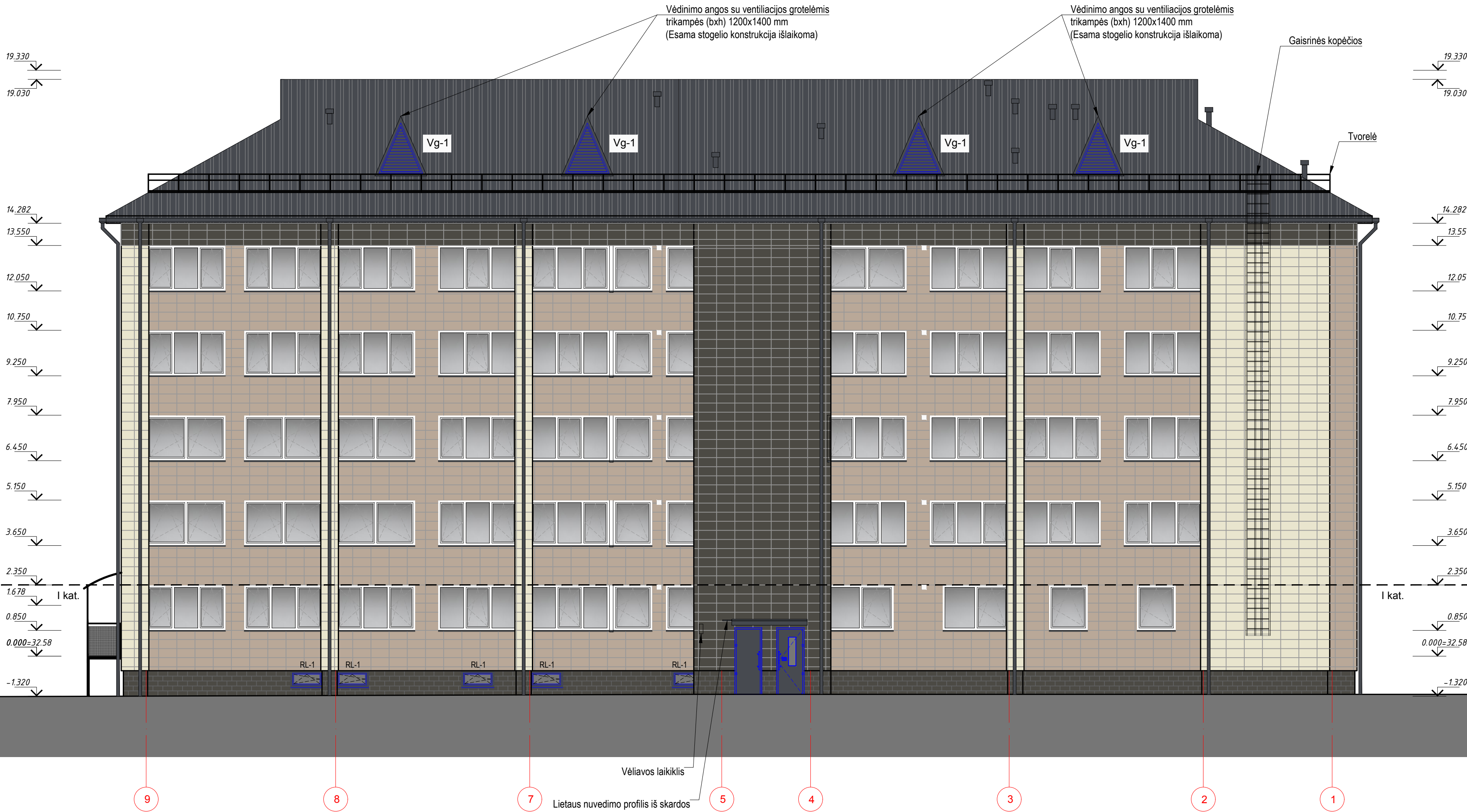
FASADAS 9-1 M 1:100
