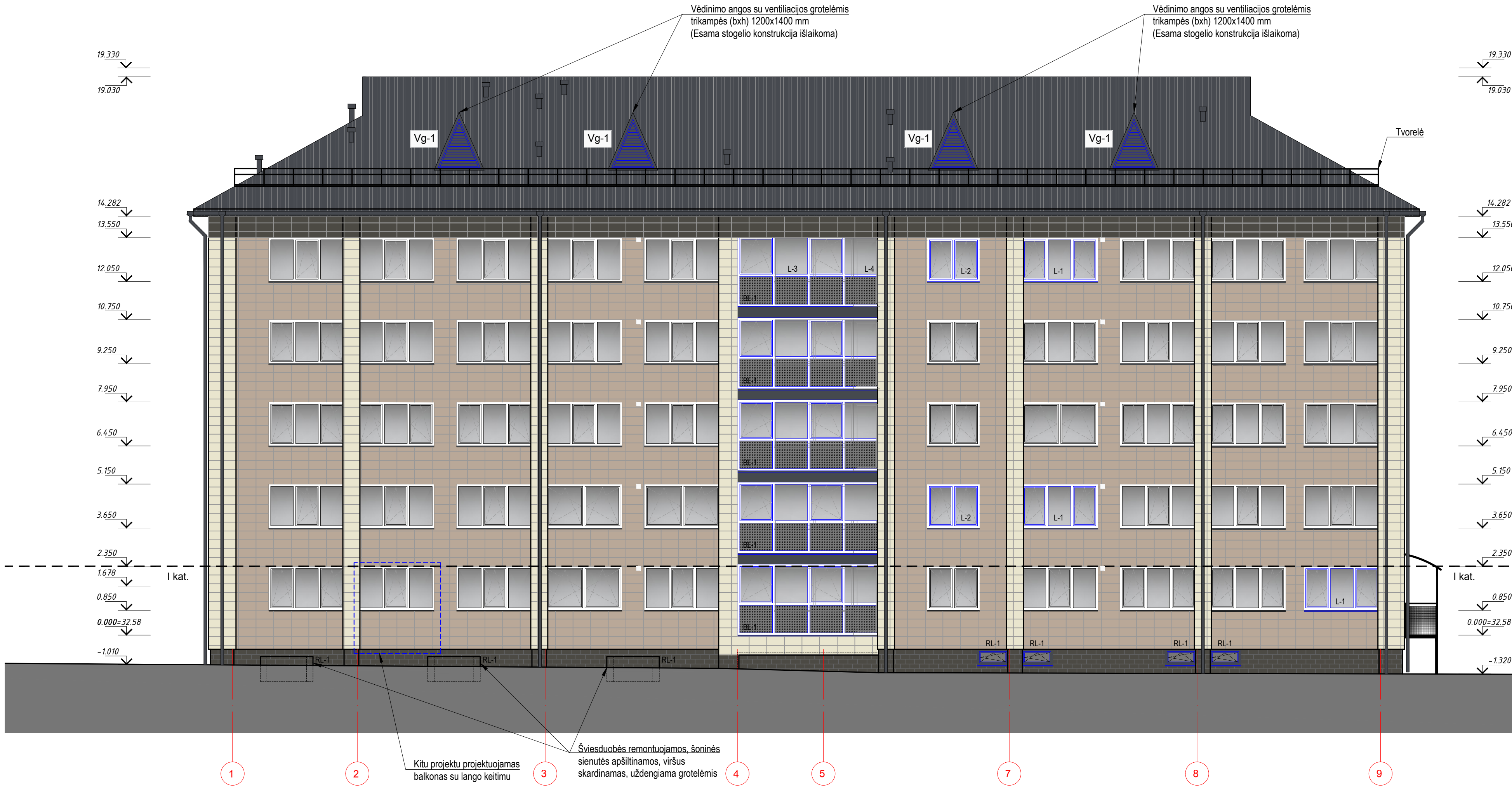
FASADAS 1-9 M 1:100
