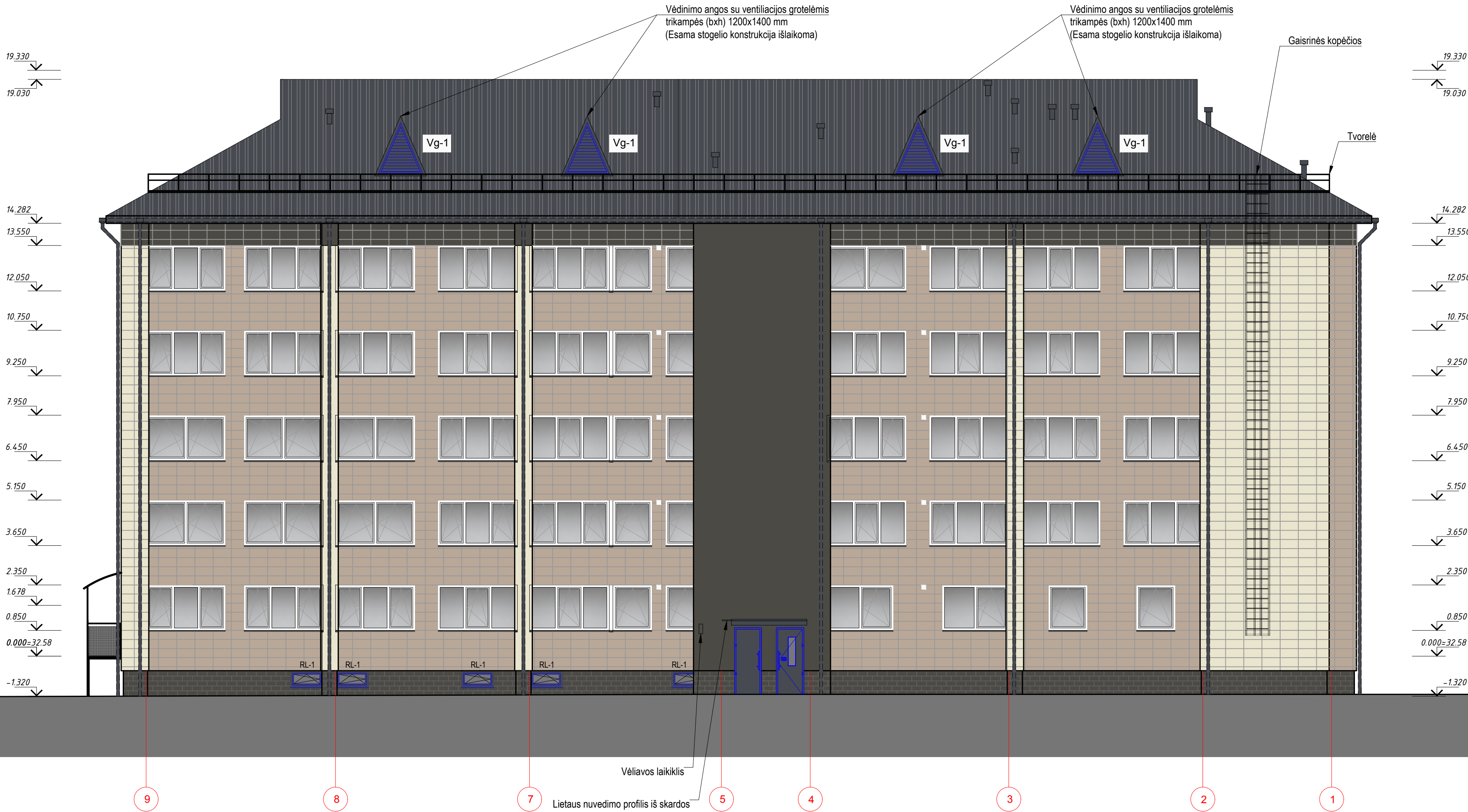
FASADAS 9-1 M 1:100
