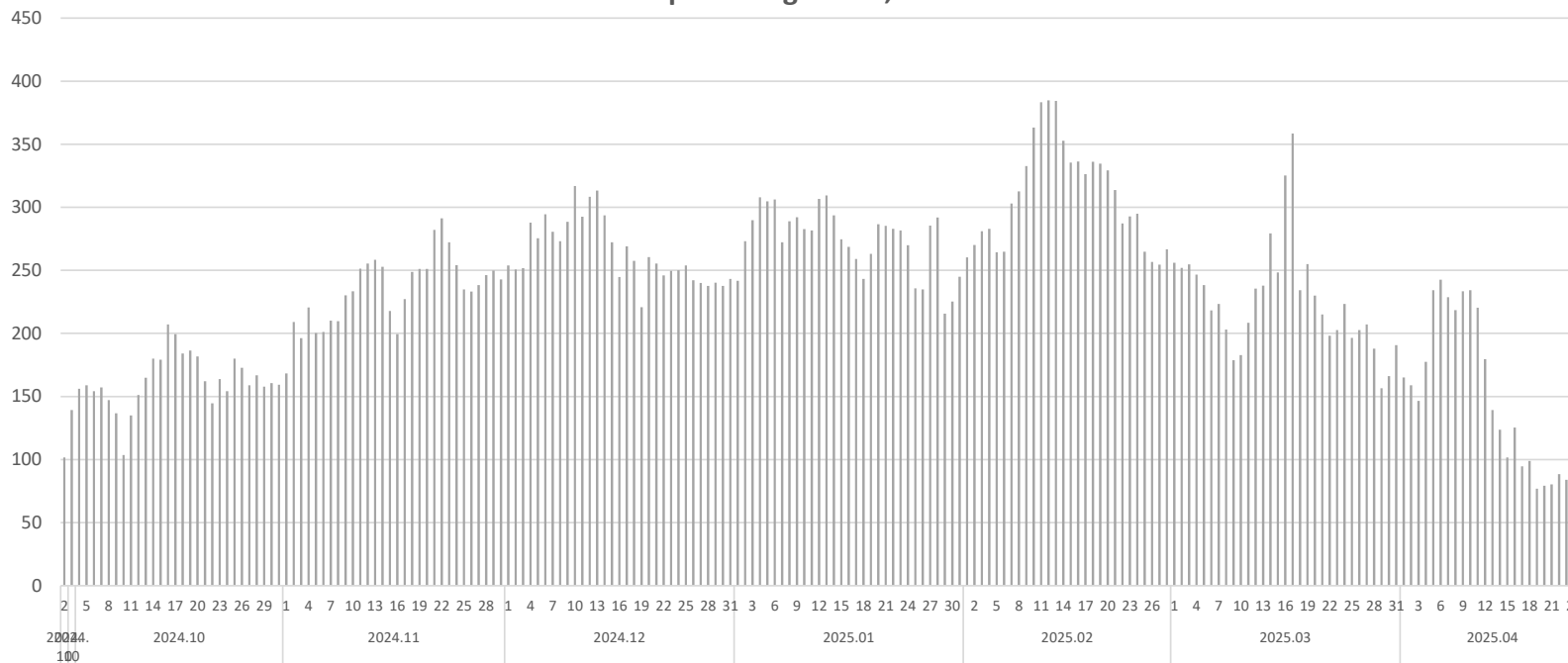
2024 - 2025 m. šildymo sezono BRK katilinės šilumos perdavimo tinklo paros vidutinio šilumos poreikio grafikas, MWh
