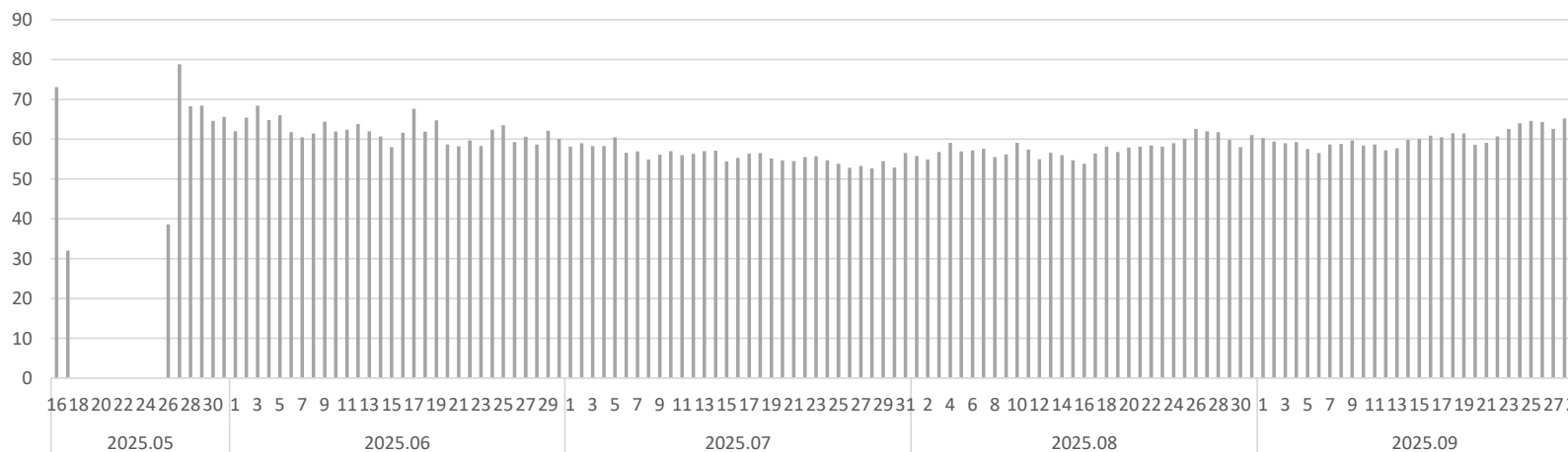
2025 m. nešildymo sezono BRK katilinės šilumos perdavimo tinklo paros vidutinio šilumos poreikio grafikas, MWh
