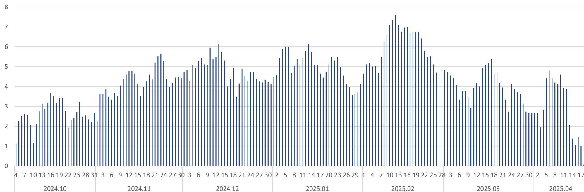
2024 - 2025 m. šildymo sezono Tauragės Dvaro katilinės šilumos perdavimo tinklo paros vidutinio šilumos poreikio grafikas, MWh
