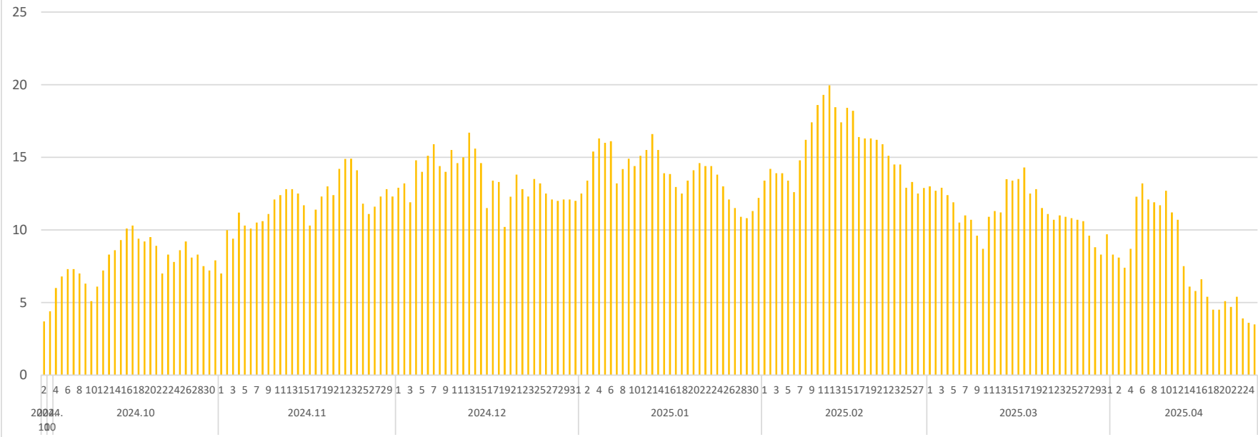
2024 - 2025 m. šildymo sezono Tarailių katilinės šilumos perdavimo tinklo paros vidutinio šilumos poreikio grafikas, MWh
