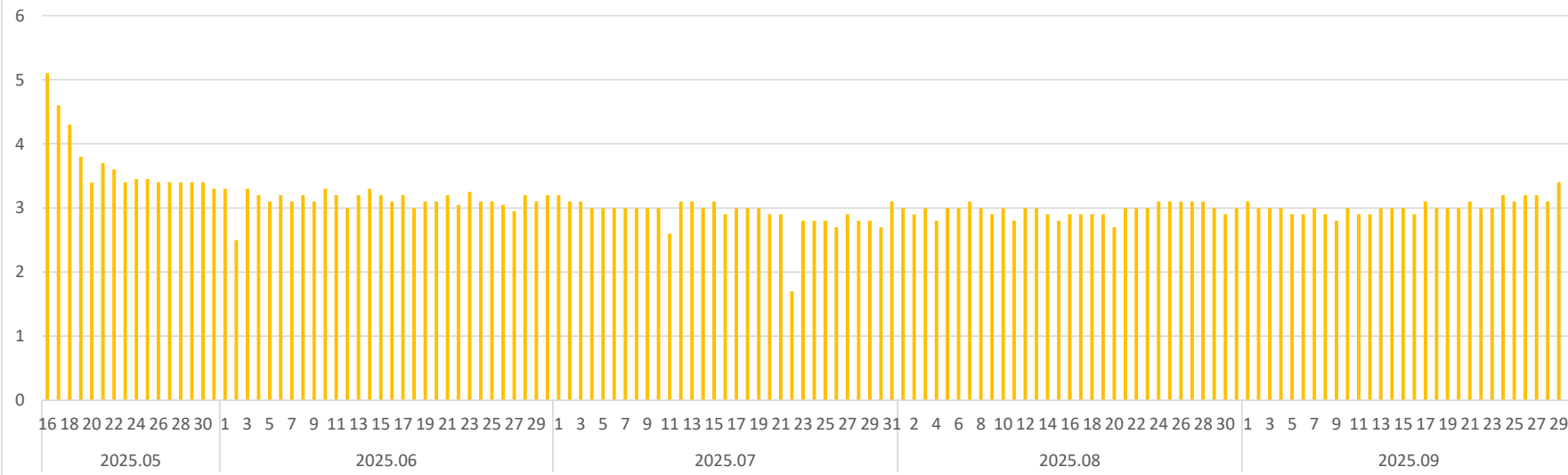
2025 m. nešildymo sezono Tarailių katilinės šilumos perdavimo tinklo paros vidutinio šilumos poreikio grafikas, MWh
